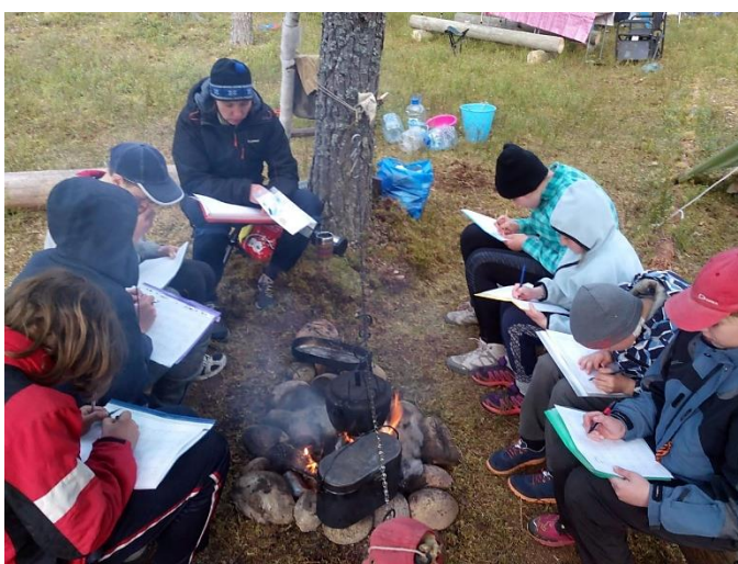
Рис.3. Настройка радиопеленгационного оборудования и разбор трассы по карте местности в походных условиях ребят из младших и старших групп
